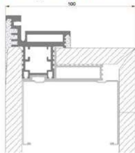
ВІД СЕБЕ ОДИН ЛИСТ ГІПСОКАРТОНУ
