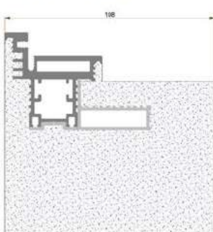
ВІД СЕБЕ ШТУКАТУРКА
